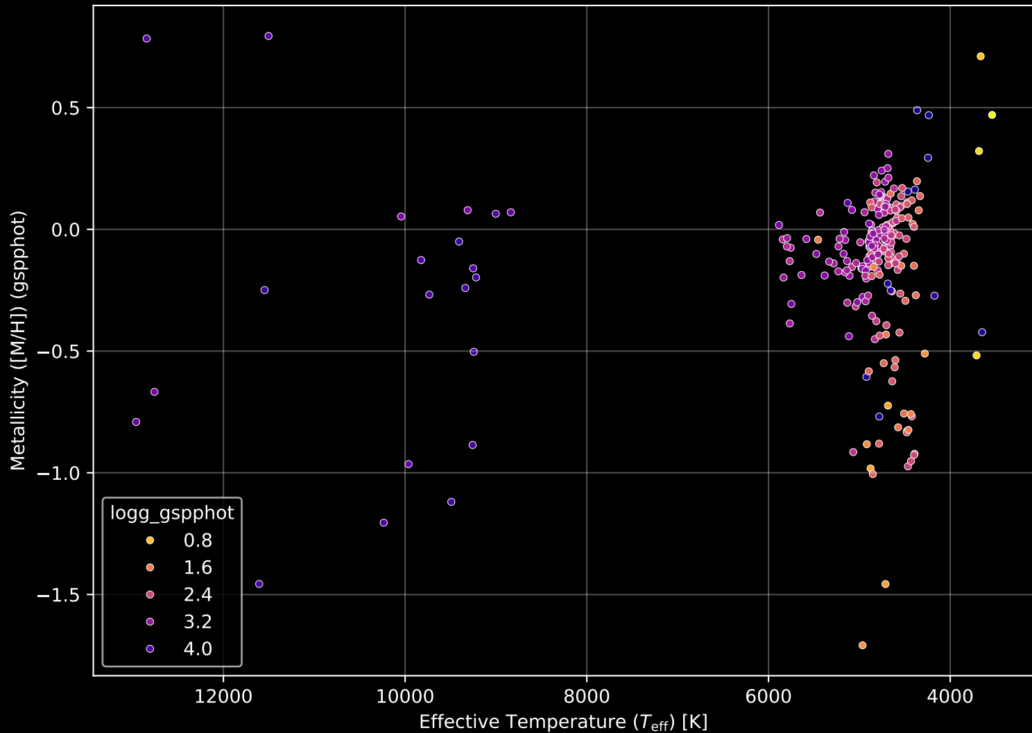
APOGEE DR17 Field: [025-12] Stellar Population Parameters (n= 254)
